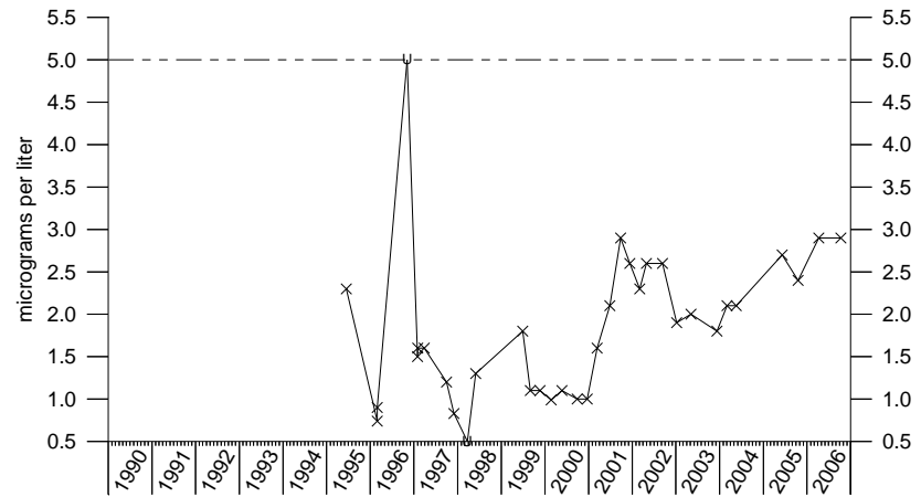
Trichloroethene IRA-6
