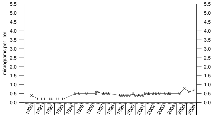
Trichloroethene IRA-1
