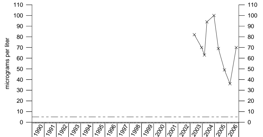
Trichloroethene IRA-22
