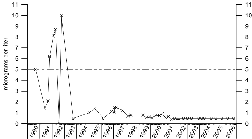
Trichloroethene IRA-1
