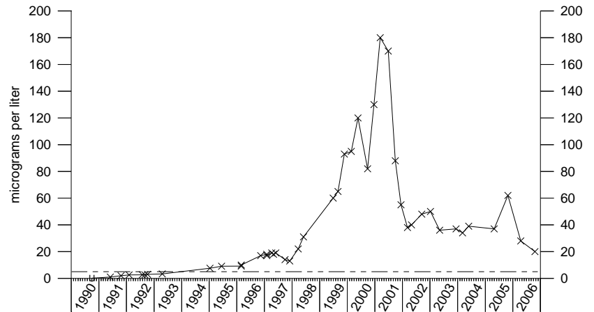
Trichloroethene IRA-2
