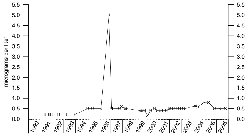
Trichloroethene IRA-5
