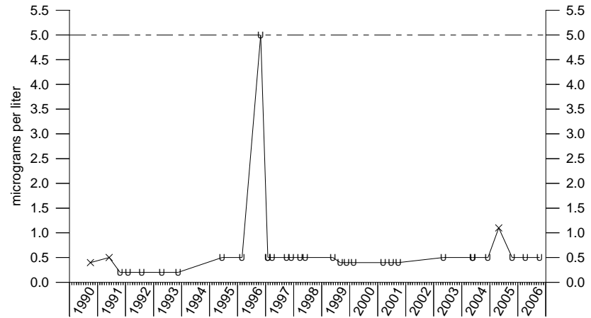
Trichloroethene IRA-6
