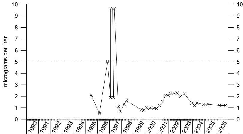
Trichloroethene IRA-9
