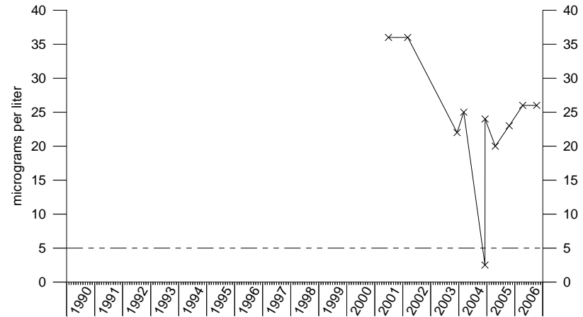
Trichloroethene IRA-17
