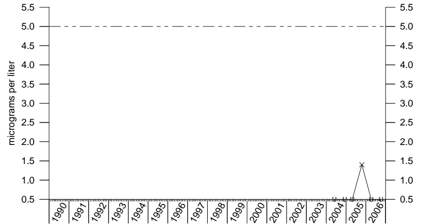
Trichloroethene IRA-26
