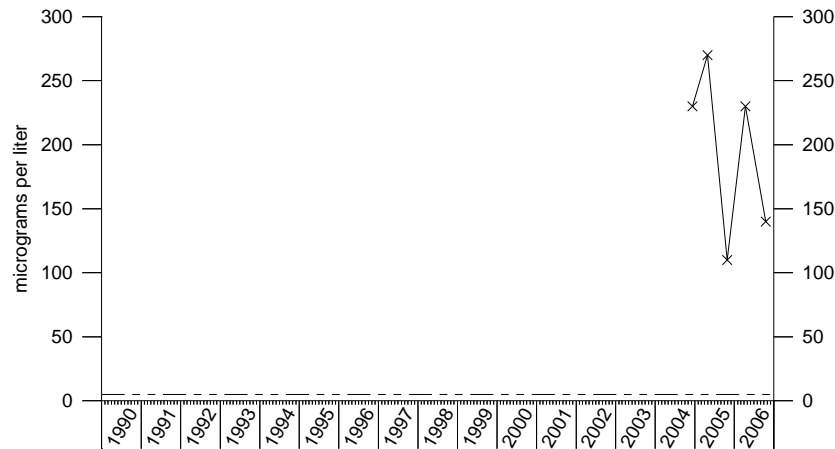
Trichloroethene IRA-30
