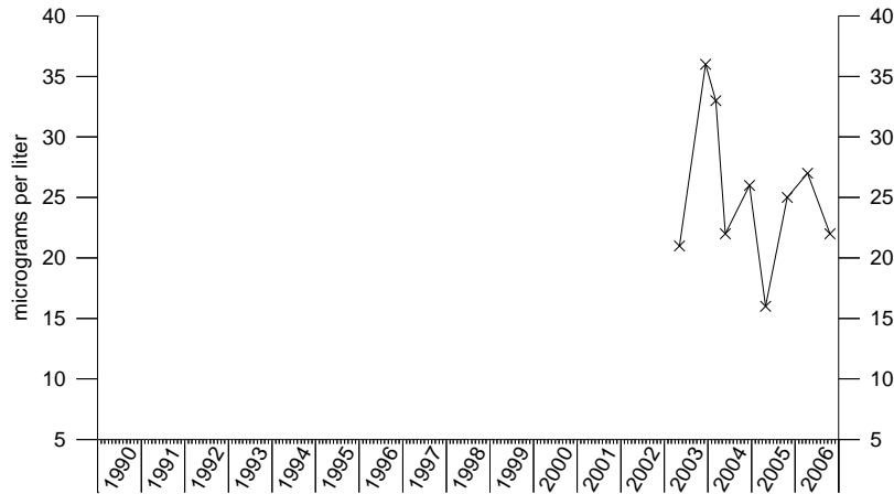
Trichloroethene IRA-25
