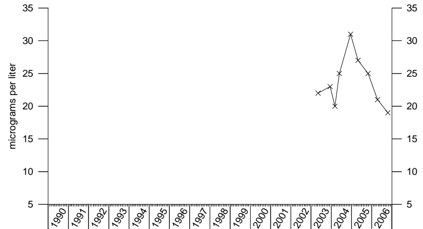
Trichloroethene IRA-14-4
