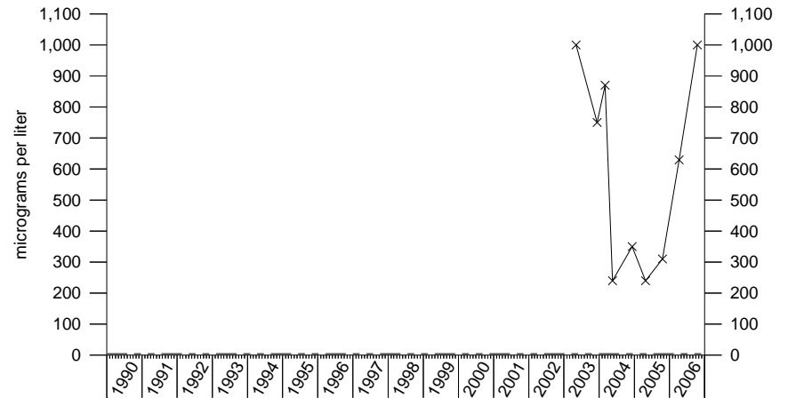
Trichloroethene IRA-17
