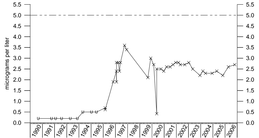
Trichloroethene IRA-2
