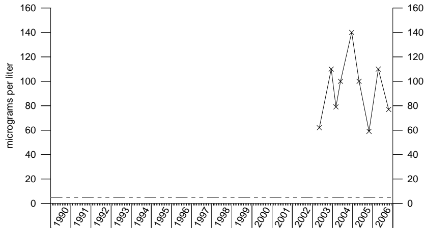
Trichloroethene IRA-21
