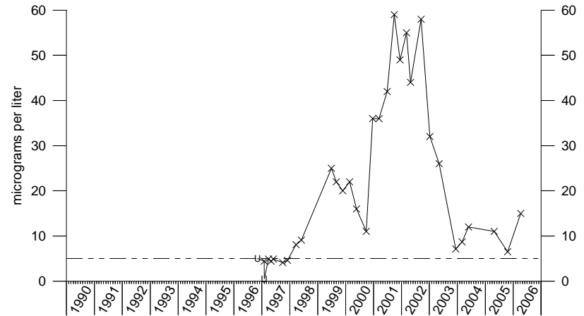
Trichloroethene IRA-8
