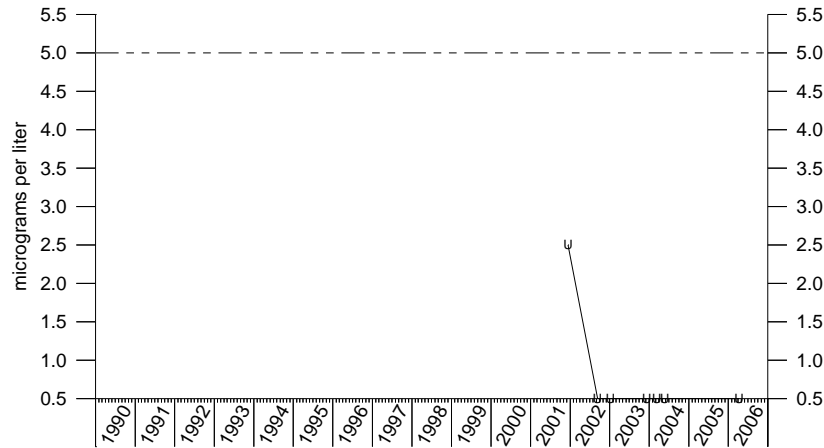
Trichloroethene IRA-16
